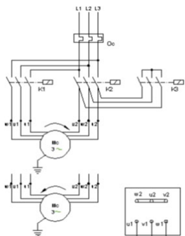
Y-D STARTER
