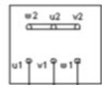
Y-D STARTER
