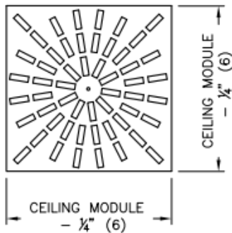
□ SQUARE ARRAY
